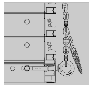
4-Strang-Gehänge (gültig für KN80-Schalungssystem)
