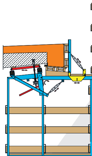
Kappenbahn
