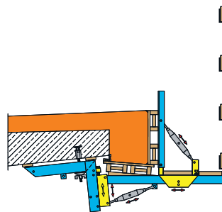
Einzelriegel
