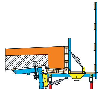
Kappenelement
